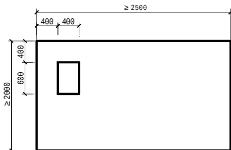
图 A.2.1 试样
