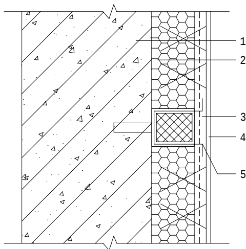
图6.5.1 机械固定系统
