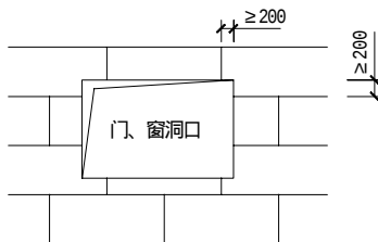
图6.1.9 (b) 门窗洞口 EPS 板排列
