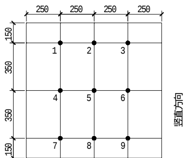
图 B.2.1 测点位置
