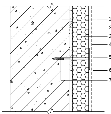
图6.1.1 EPS 板薄抹灰系统
