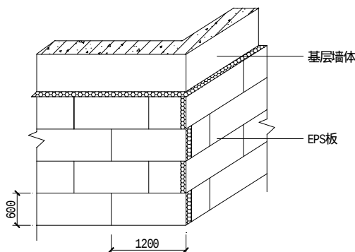
图6.1.9 (a) EPS 板排版图
