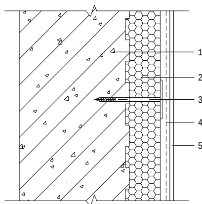
图 6.3.1 无网现浇系统
