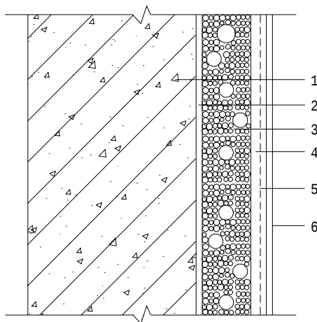
图6.2.1 保温浆料系统
