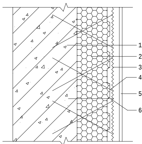
图6. 4. 1 有网现浇系统
